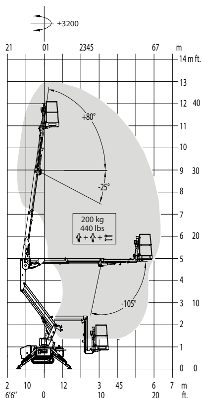
▲ Рабочая высота и вылет
